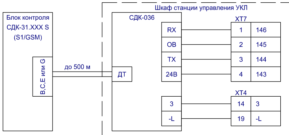
Рис. 2. Подключение к станциям типа УКЛ
