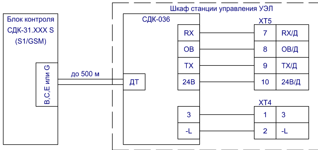
Рис. 1. Подключение к станциям типа УЭЛ
