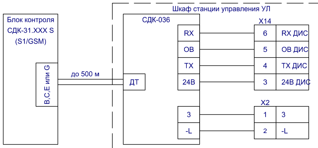
Рис. 3. Подключение к станциям типа УЛ
